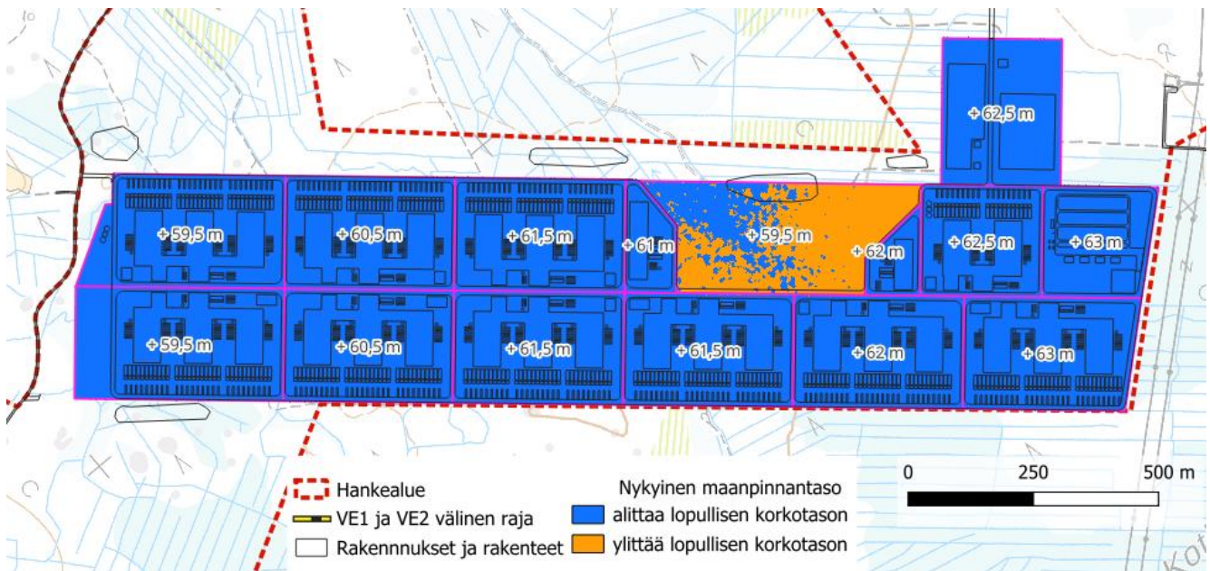
Kuva 15-1. Kuvassa havainnollistetaan mitä osa-alueita joudutaan täyttämään (siniset) ja laskemaan (oranssit), jotta maanpinta saadaan haluttuun korkotasoon. Kuva perustuu Maanmittauslaitoksen avoimeen laserkeilausaineistoon sekä alustavaan, optimoimattomaan, tasaussuunnitelmaan. Sisältää Maanmittauslaitoksen avointa aineistoa (3/2026).
