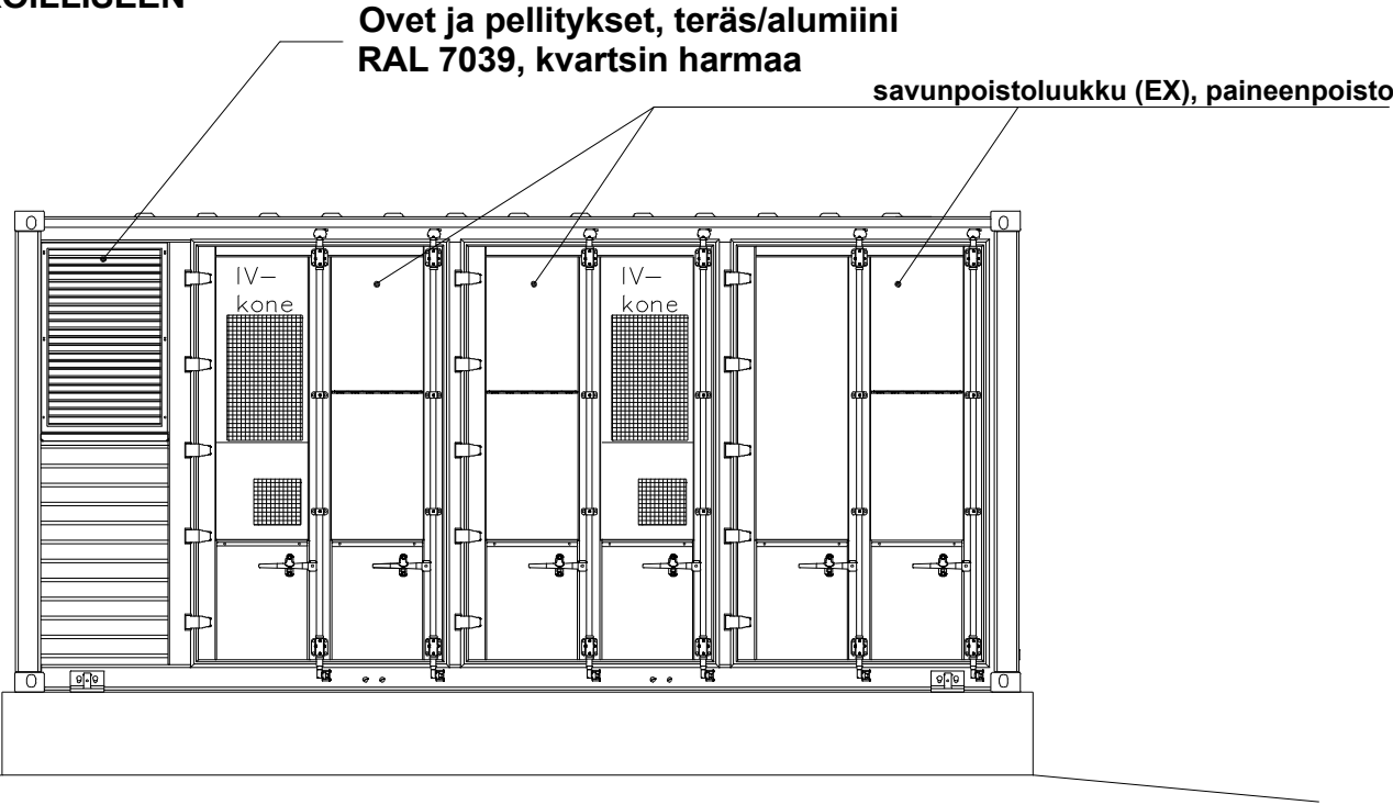
JULKISIVU KOILLISEEN
