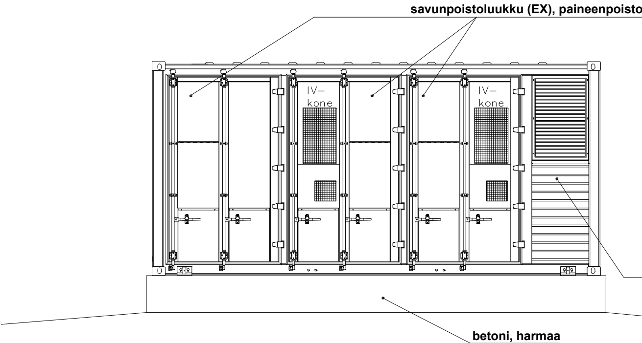
JULKISIVU LOUNAASEEN
