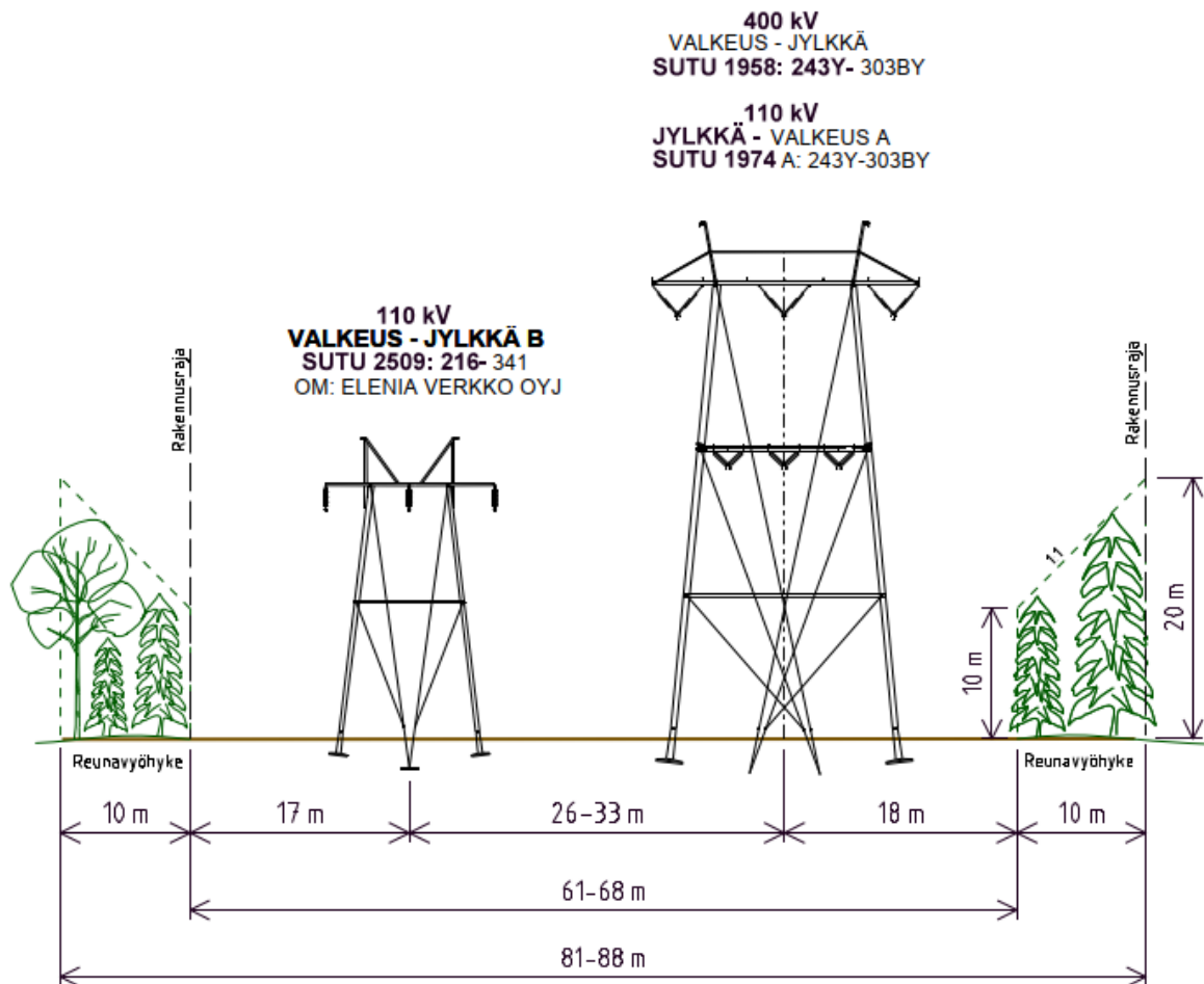
Kuva 36. Poikkileikkaus Valkeuden sähköasemalle liittyvistä nykyisistä voimajohdoista. Kuva: Fingrid.
